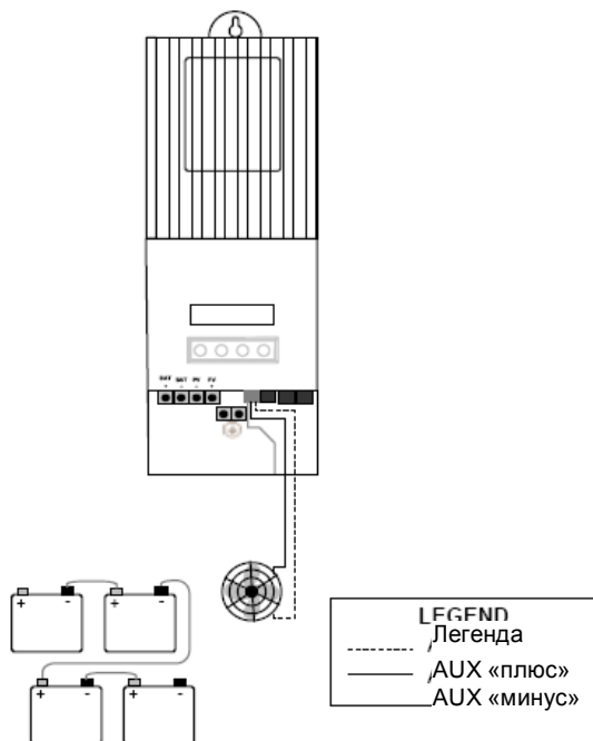
Рисунок 2-11 Подключение вентилятора к дополнительному выходу
