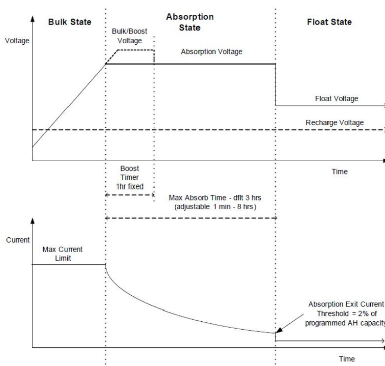
Рисунок 1-4 Трехстадийный цикл зарядки батарей а
