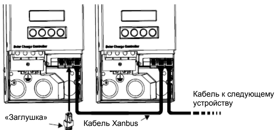
Рисунок 2-13 Конфигурация Xanbus
