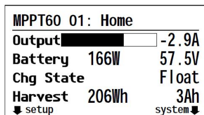
Рисунок В-8 Главный экран (Home Screen)
