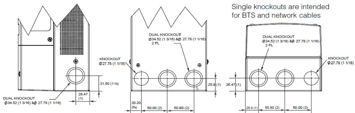
Рисунок 2-4 Монтажные отверстия для кабелей
