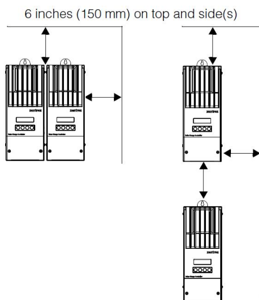
Рисунок 2-1 Минимальные требования к зазорам
