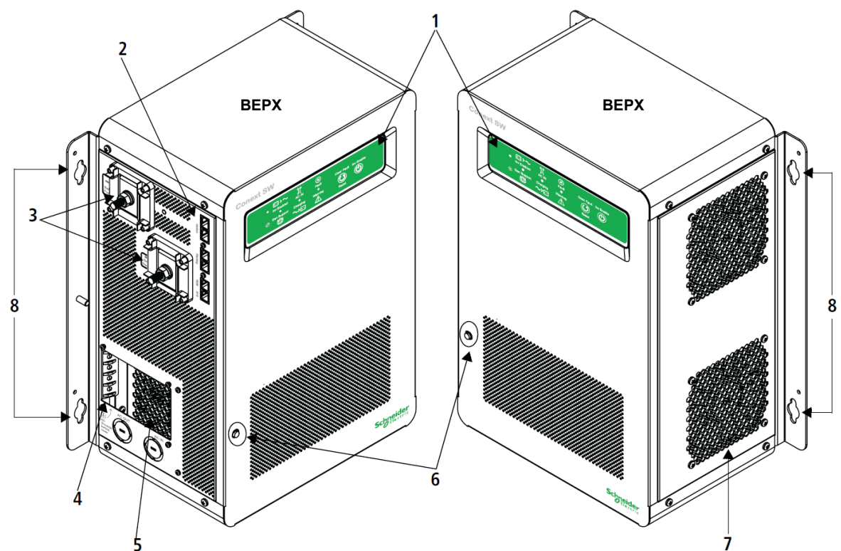
Рисунок 2-2 Передняя и боковая панели Conext SW
