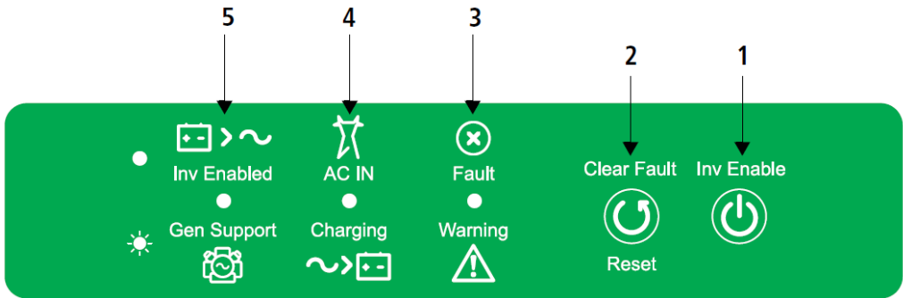
Рисунок 2-3 Светодиоды передней панели
