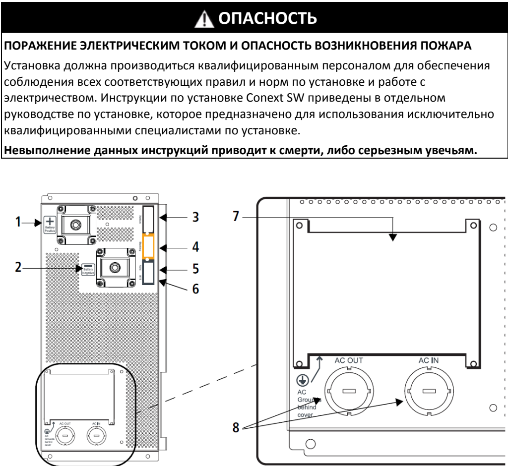
Рисунок 2-4 Терминалы постоянного и переменного тока
